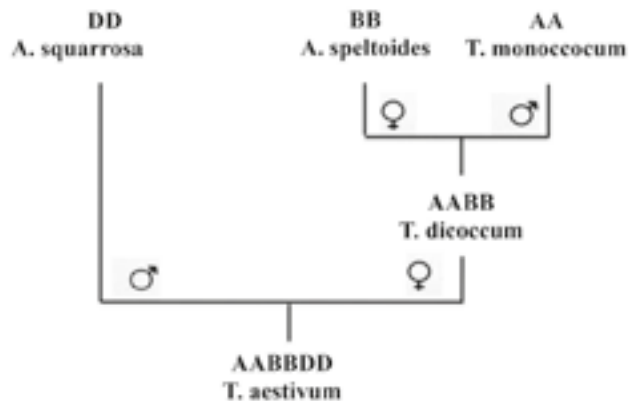
Esquèma dels dos crosaments naturals a l'origina del blat dur e del blat tendre, d'après l'idrolisi dels ADN cloroplastics e mitocondrials (d'hereditat mairala), per una enzima de restricció (6).
